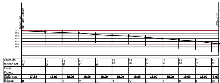
Perfil longitudinal Esc: 1/1000
